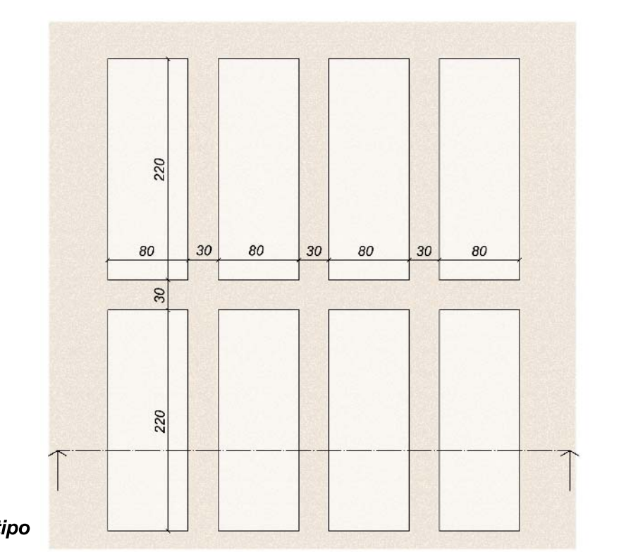
SCHEMA TIPO INUMAZIONI IN CAMPO COMUNE
