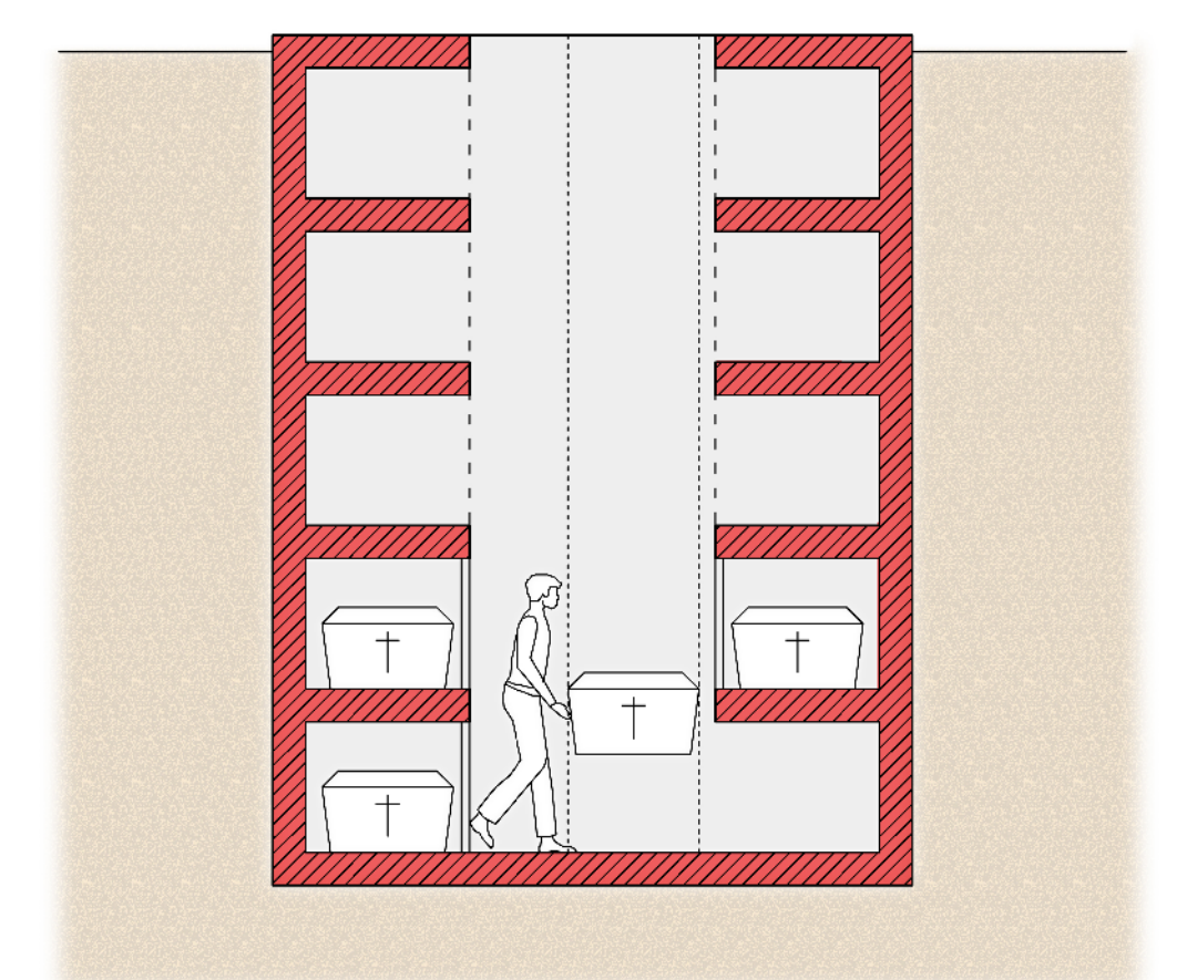
SCHEMA SEZIONE TIPO INUMAZIONI IN TOMBA
